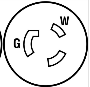
Receptacle
